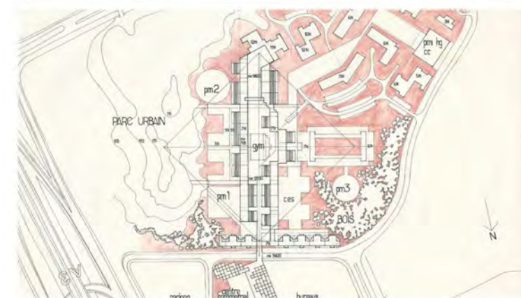
900 logements. Plan-masse. Échelle au 1/2000e. Cité de l'architecture & du patrimoine/Musée des Monuments français. 2017
